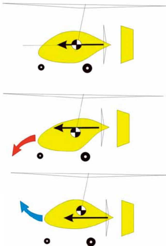
螺旋桨推力轴相对于重心的位置（上面和下面）会影响旋翼机的俯仰稳定性
